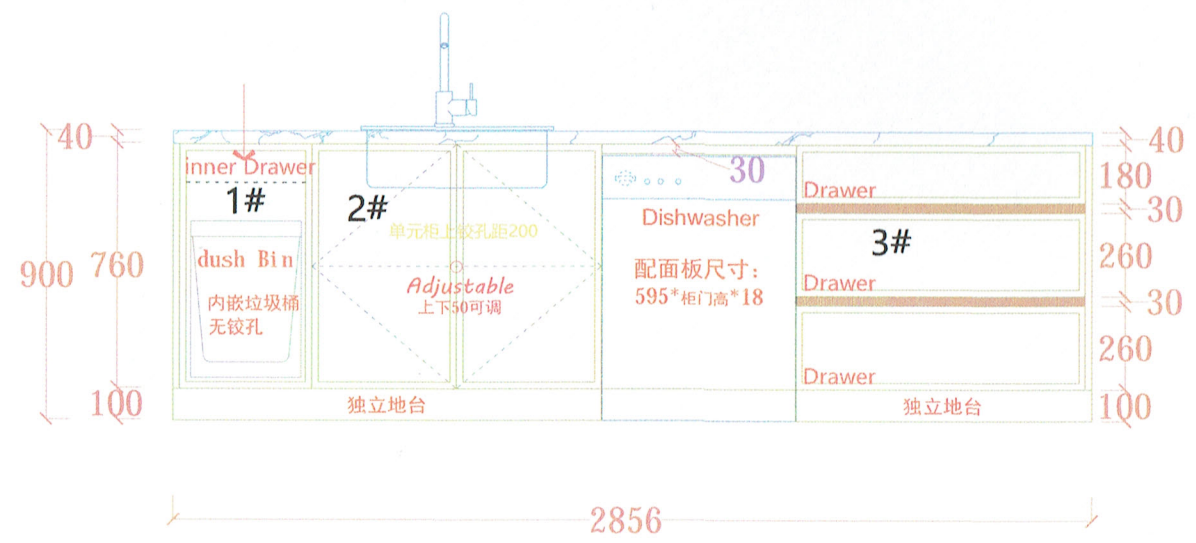
ELEVATION A
