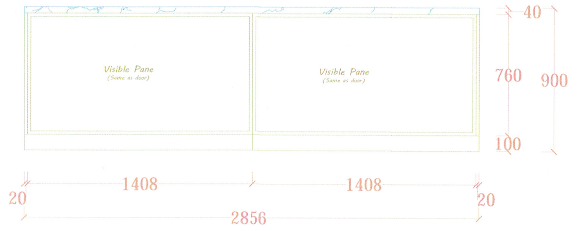
ELEVATION B
